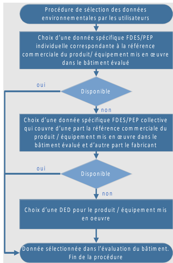
Figure 1: Logigramme pour la sélection des données environnementales dans le cadre de la démarche PEBN/RE2020
