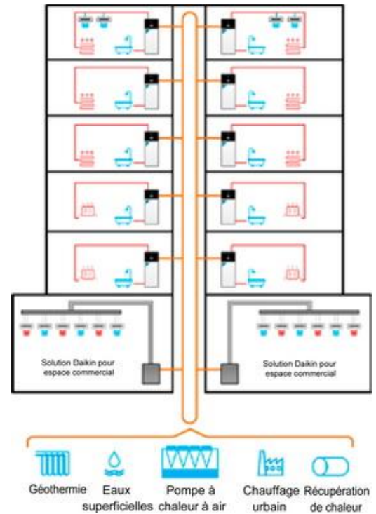
Représentation de la solution (DAIKIN)
