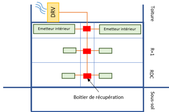
DRV chauffage seul avec un boîtier intermédiaire par étage
