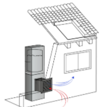
PAC intérieure : positionnée à l'intérieur du logement connecté à l'extérieur par une grille droite
