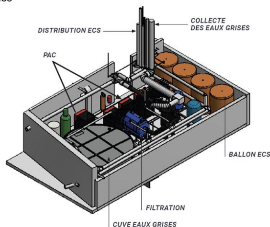
PAC sur eaux grises
