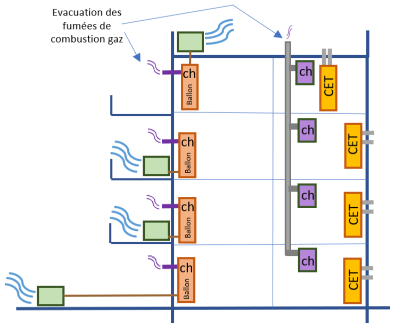
Représentation des différentes solutions d'intégration de PAC hybride (à gauche) et CET + Chaudière gaz (à droite)
