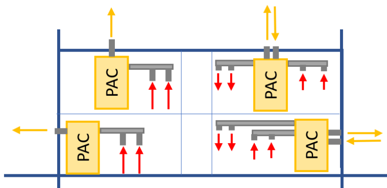
Représentation des différentes solutions d'intégration de PAC sur air extrait avec ventilation simple flux (à gauche) PAC sur air extrait avec ventilation simple double flux (à droite)
